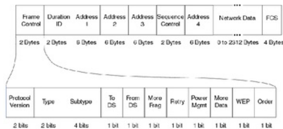
Figure-9. 802.11 MAC header(Savvius Inc.)
